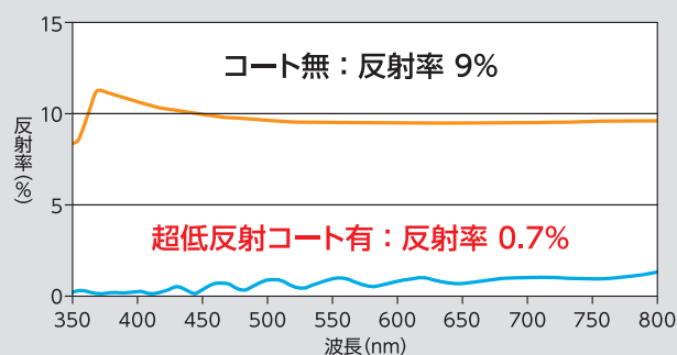
低反射コートによる反射率の違い
